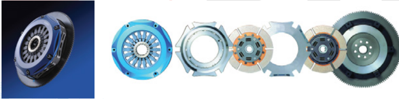
Twin Metal Clutch System : 667 022 TP - $2526 msrp
