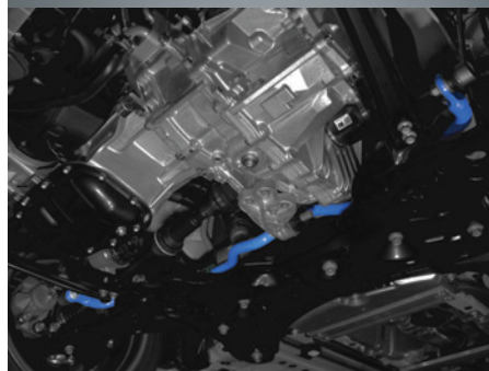
Front Sway Bar : 26mm OD / Solid - 1A1 311 A26 - $374 MSRP - 4996 3380 62239
